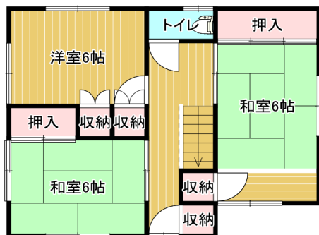
2階平面図
